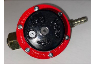
Ayarlanabilir Bütan Regülatörü
