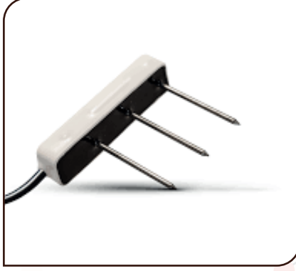
TEROS-10 (Nem) TEROS-11 (Nem + Sıcaklık) TEROS-12 (Nem + Sıcaklık + EC)
