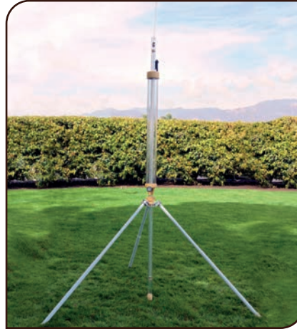
Guelph Permeametre Aardvark Permeametre
