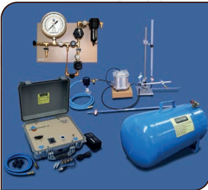
LAB1250 (Vakumlu Sistem)
