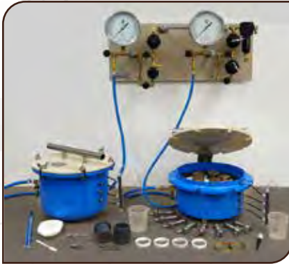
1500FS - 1600F1 (Basıncılı Tencere)
